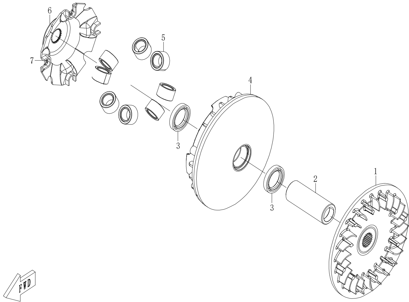
E16 KL500-B-051000主动轮组合（附图）PRIMARY SHEAVE
