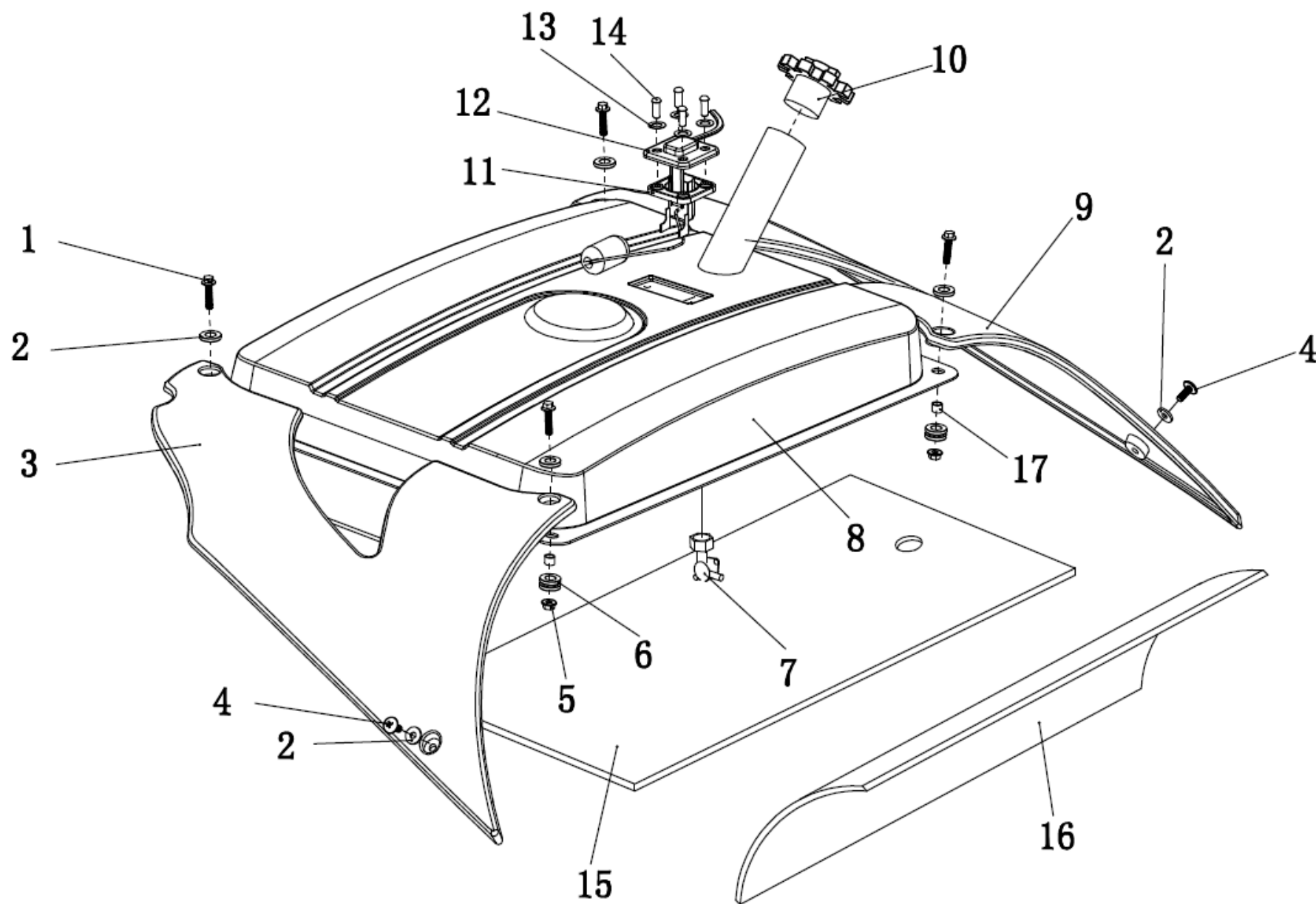
F16 油箱总成 FUEL TANK
